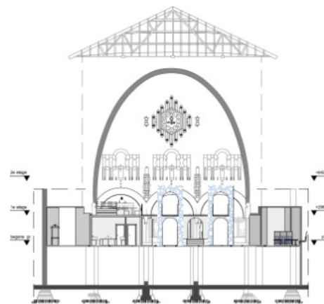
doorsnede E-E
