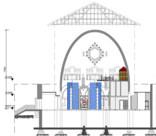
doorsnede D-D
