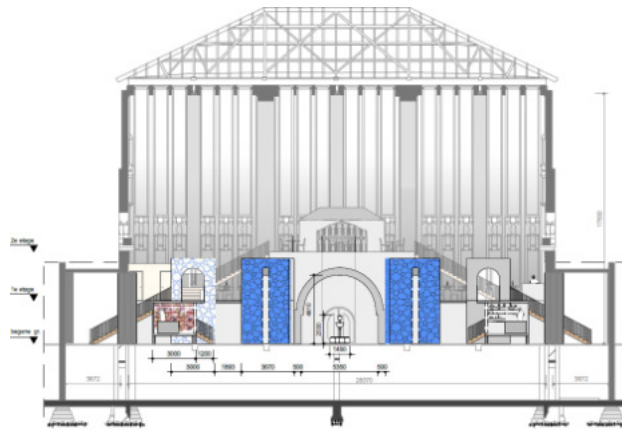
doorsnede B-B
