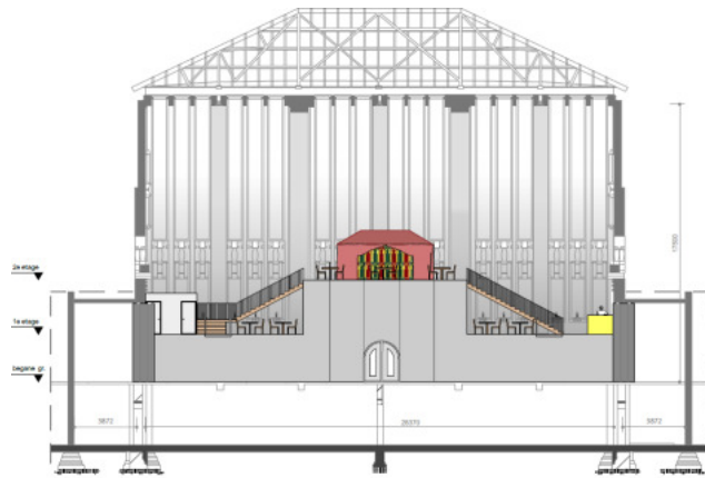
doorsnede A-A
