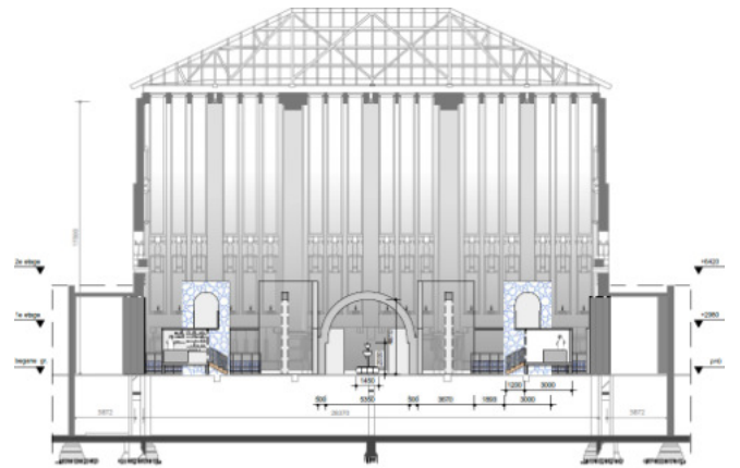
doorsnede C-C
